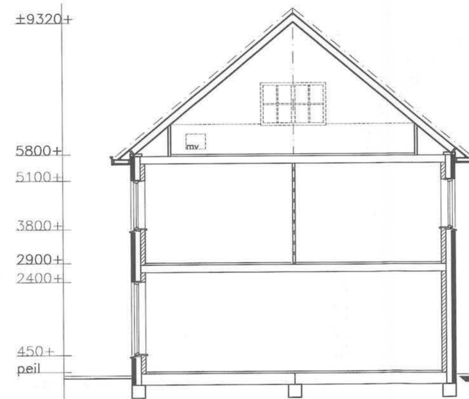
doorsnede
