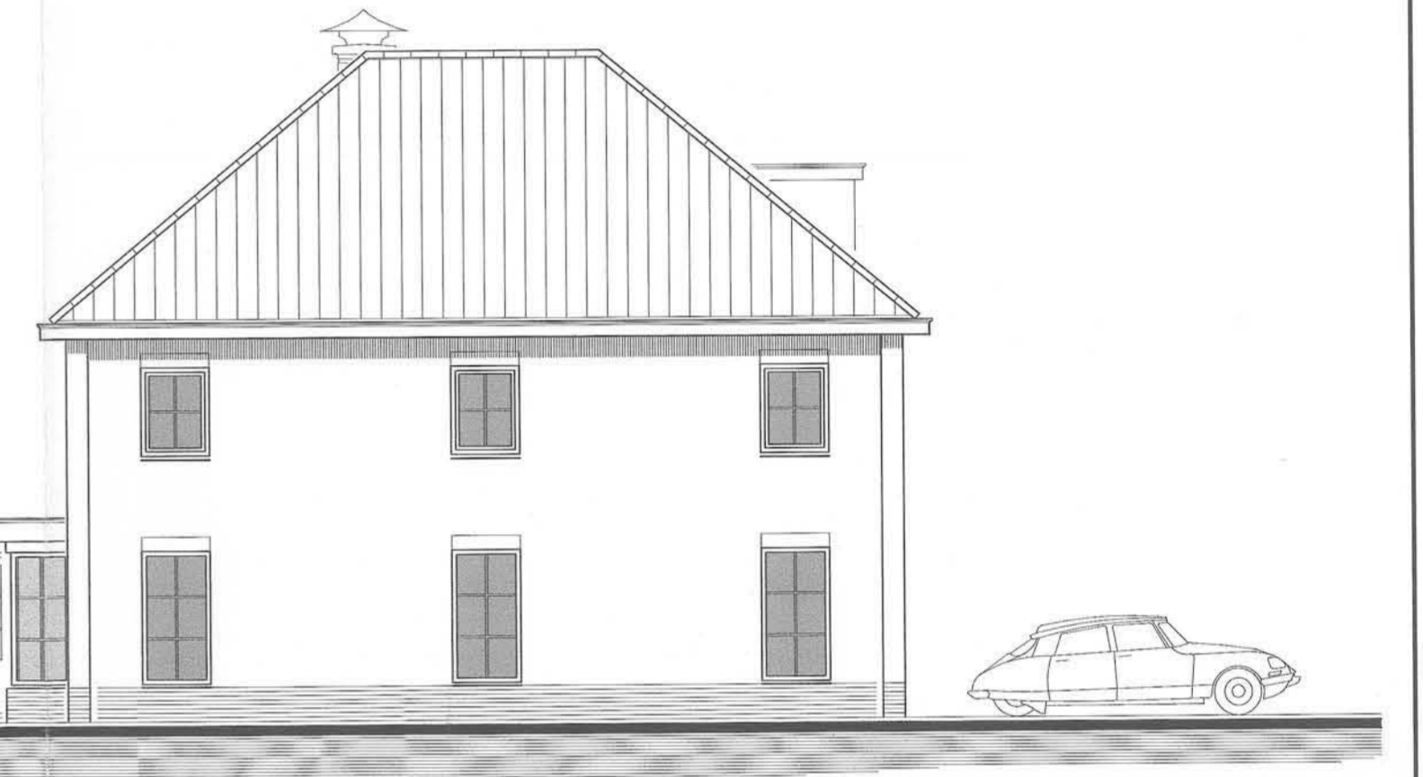
linker zijgevel
