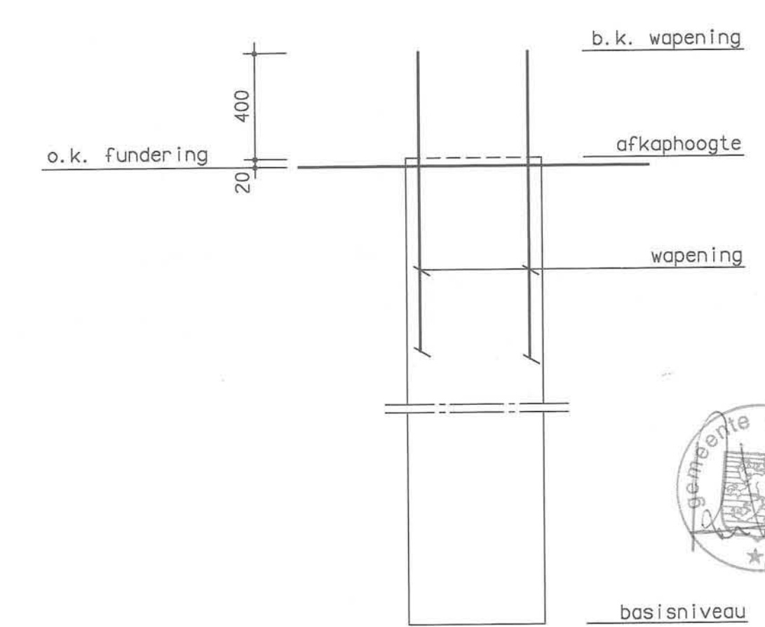
Algemeen detail heipalen
