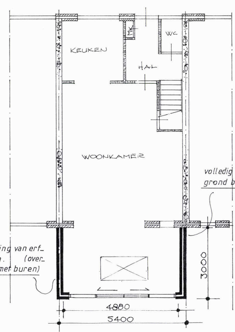
gew. plattegrond
