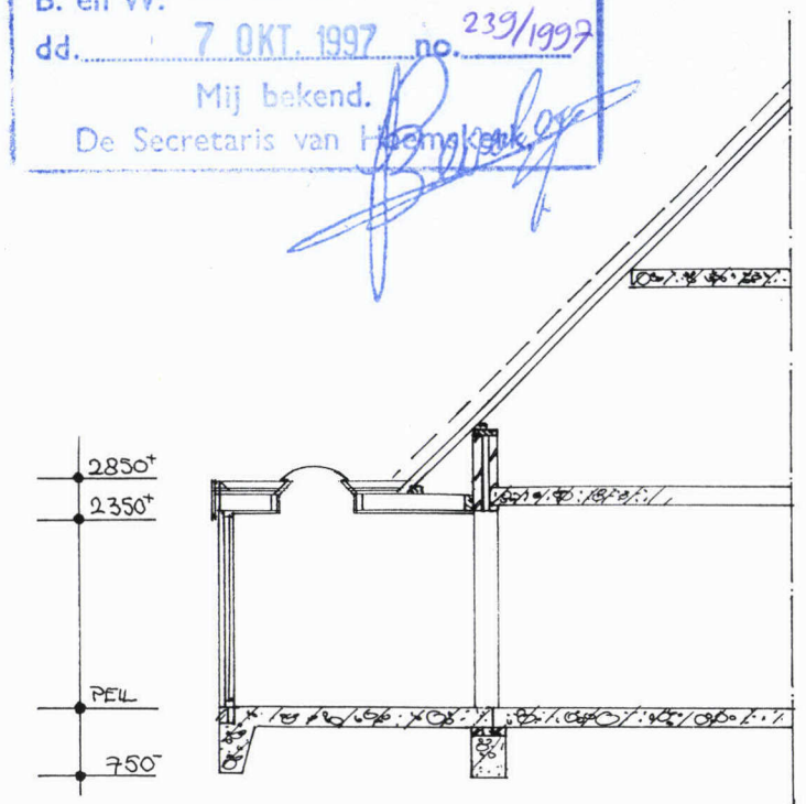
gew. doorsnede
