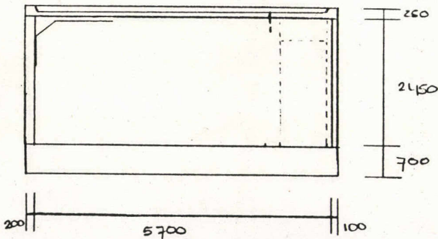
Lengte doorsnede
