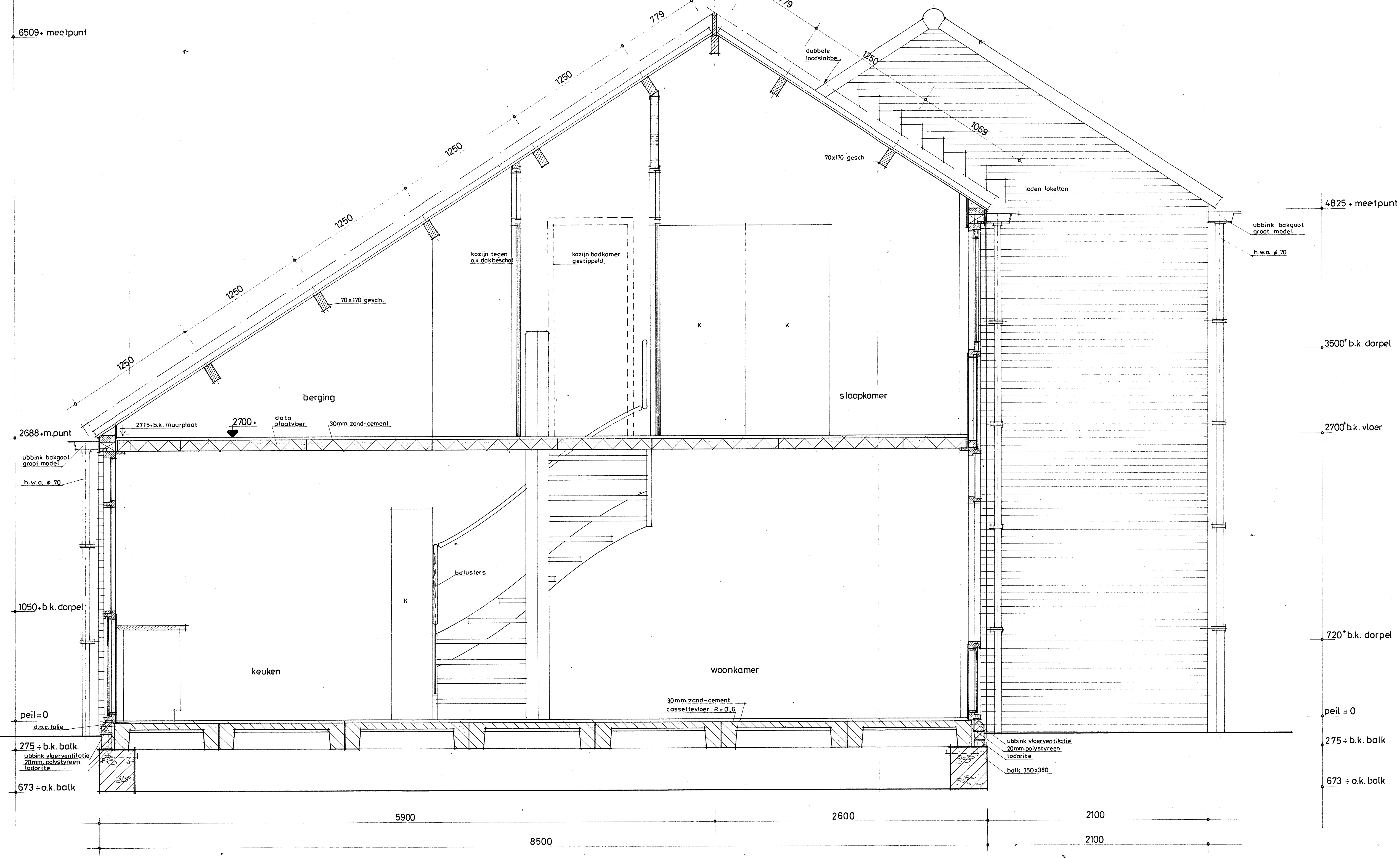
DOORSNEDE II-II
