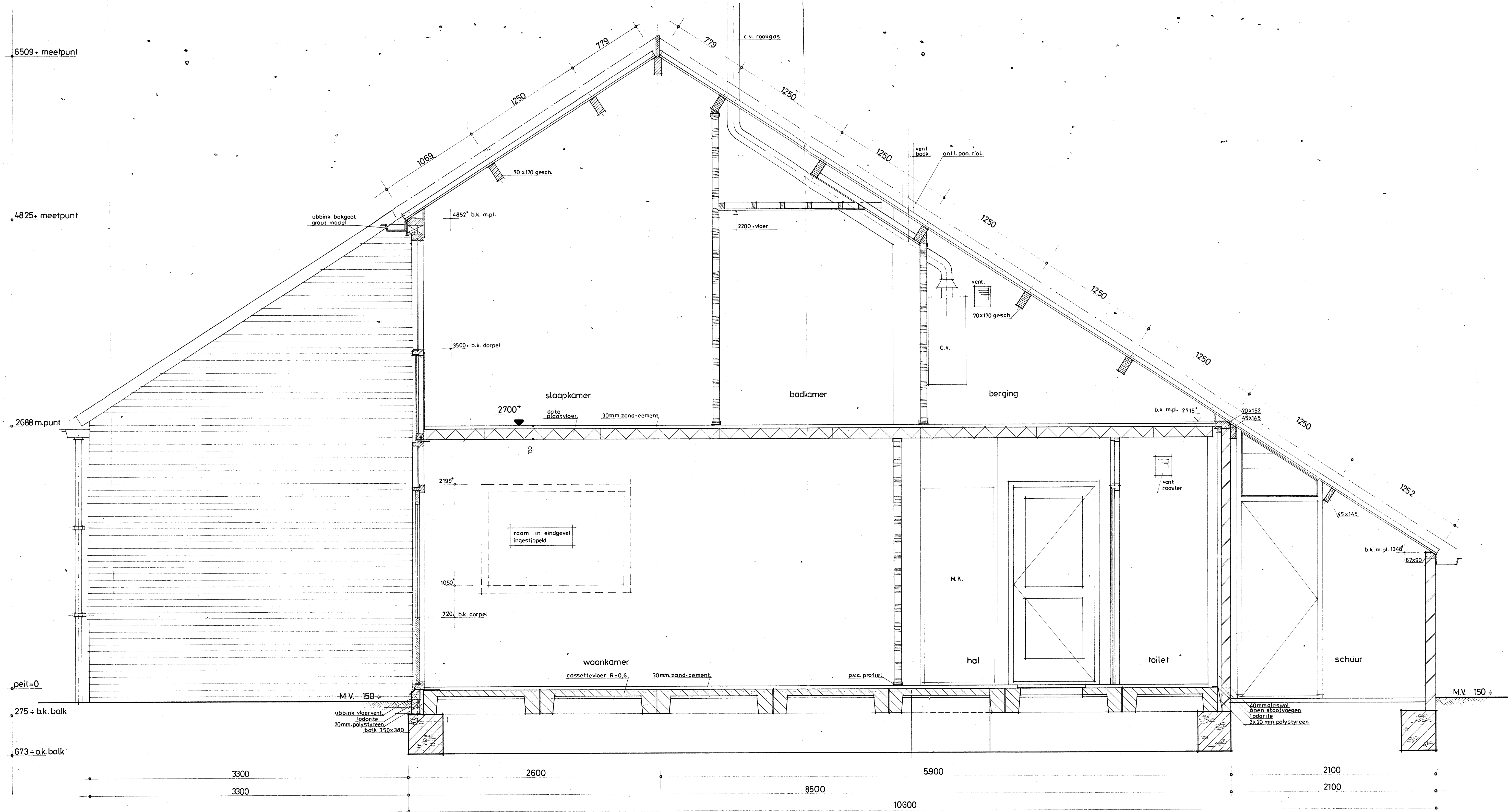
DOORSNEDE I-I
