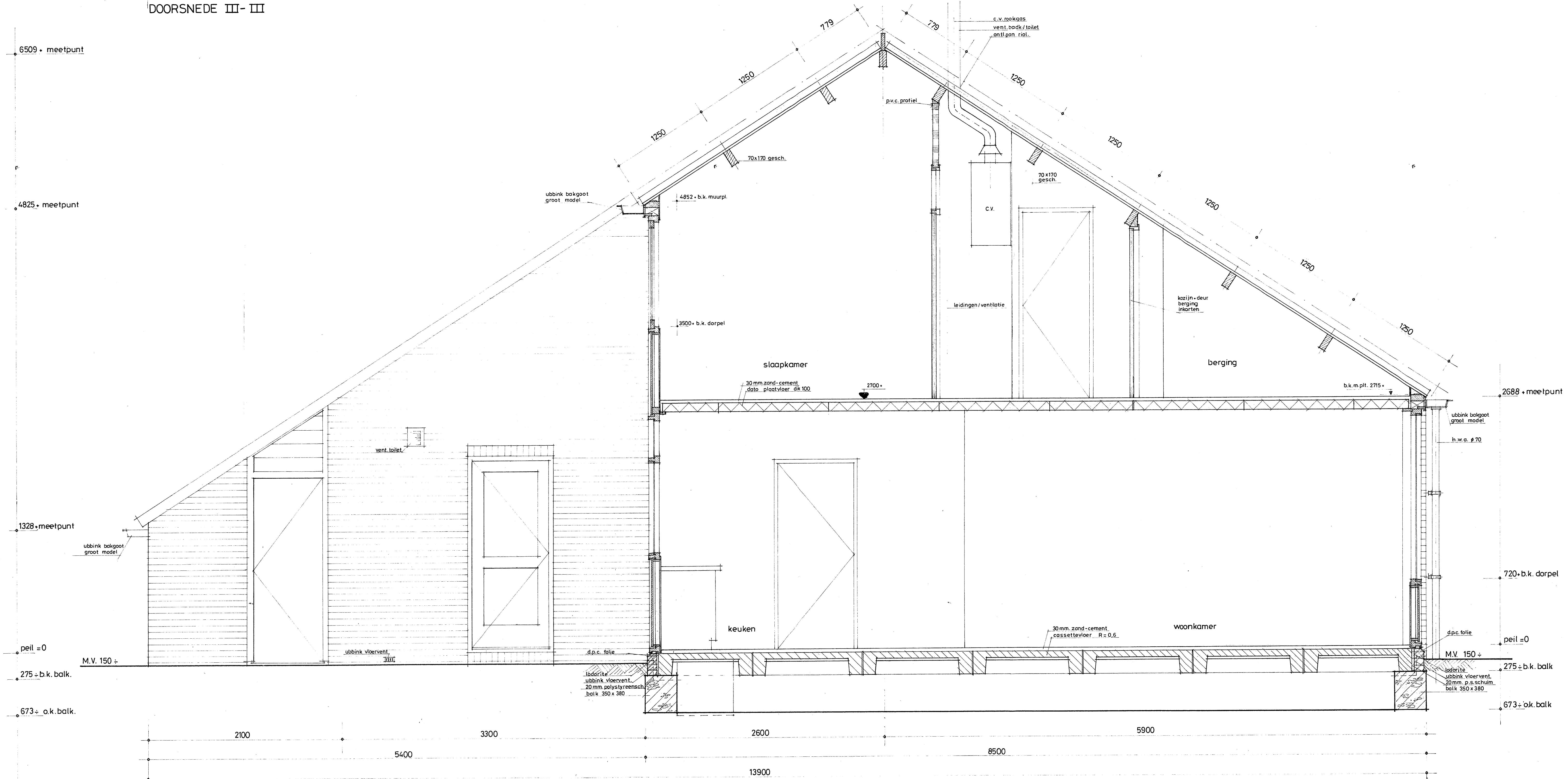
DOORSNEDE IV-IV
