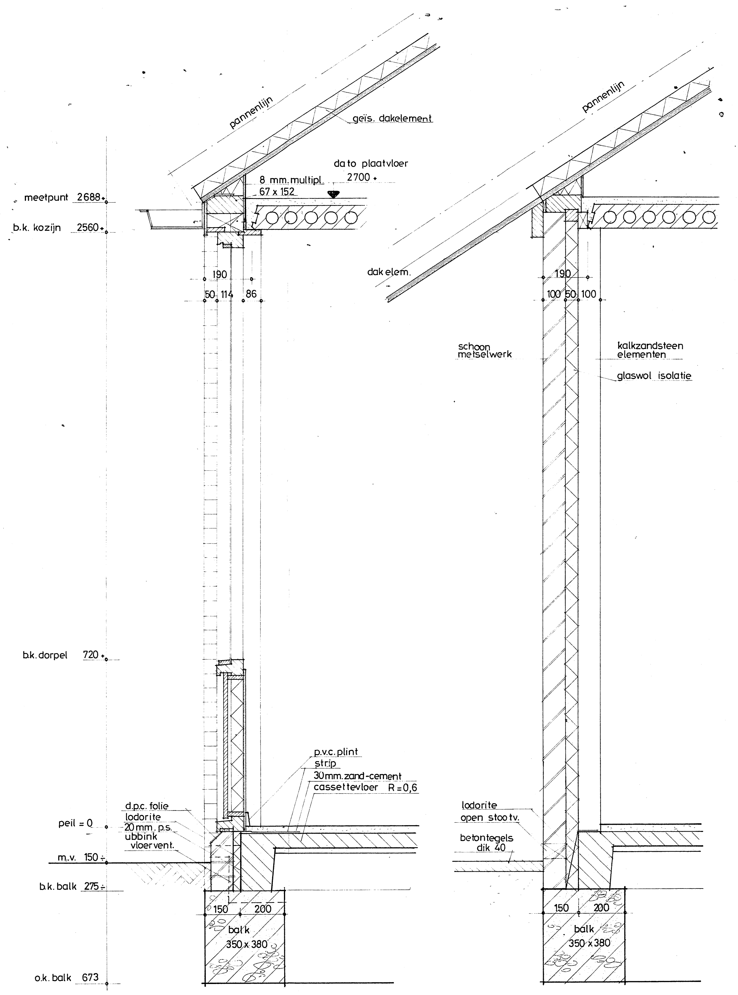
DOORSNEDE IV
