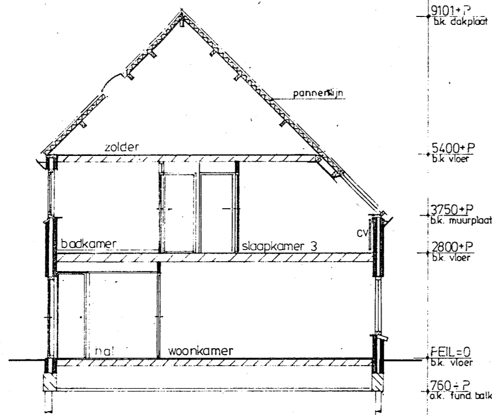
Doorsnede bestand
