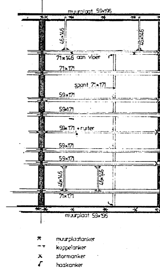
Kapplan bestand
