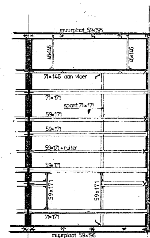
Kapplan nieuw
