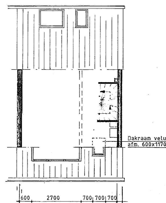
Zolder nieuw
