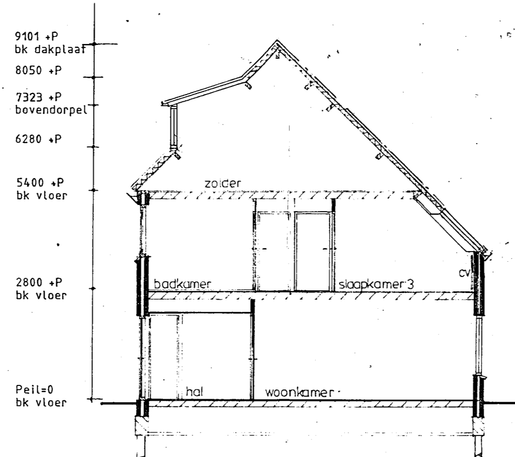
Doorsnede nieuw
