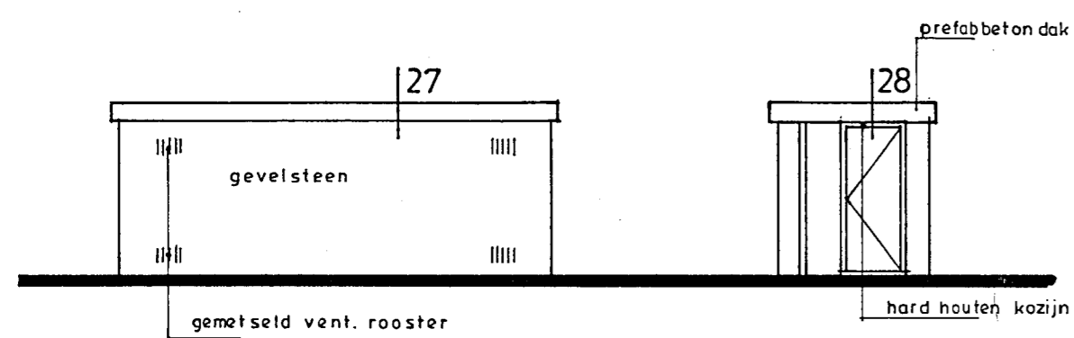
POORT c.q. TUINGEVEL DUBBELE LOSSE BERGING.
