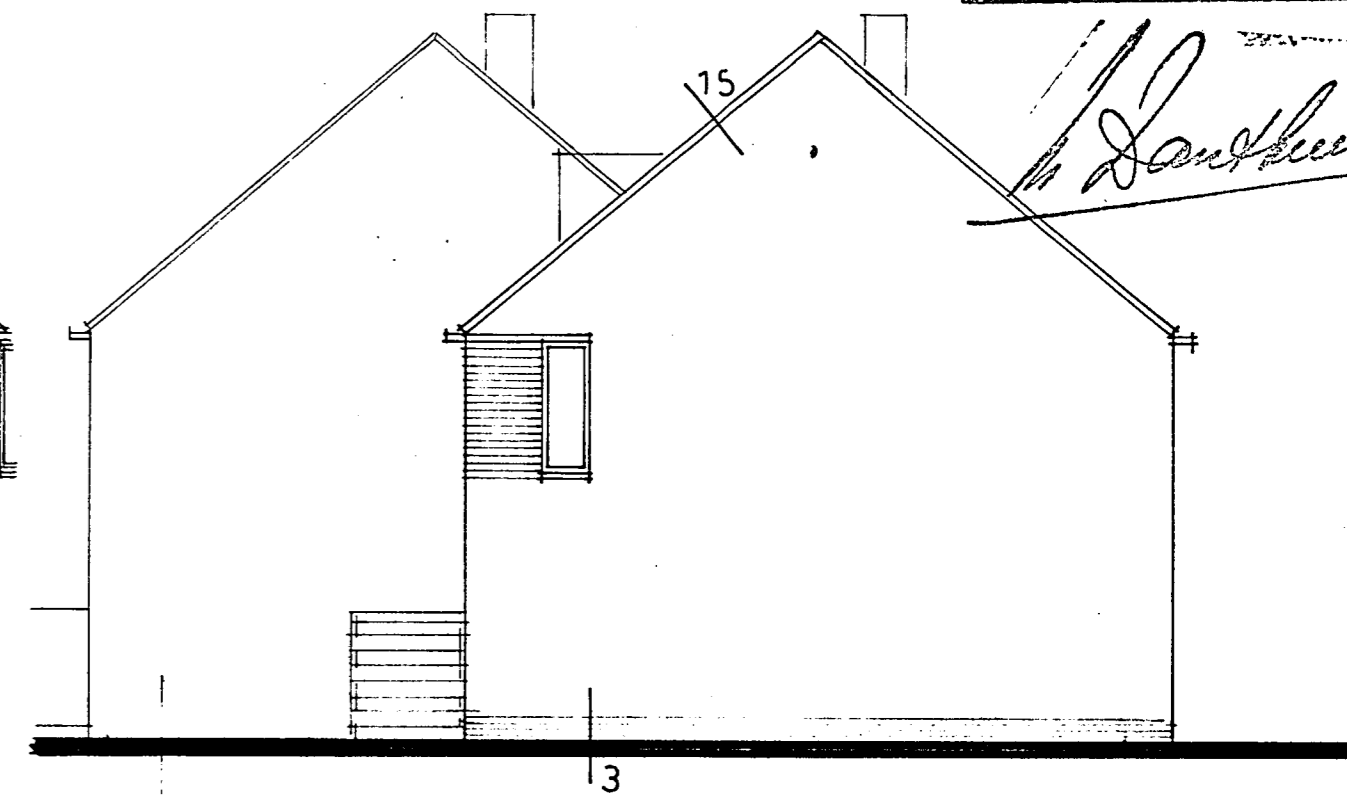
KOPGEVEL ENTREEZIJD - raam vervalt bij aansl. op garage en bij woningnrs. 23, 38
