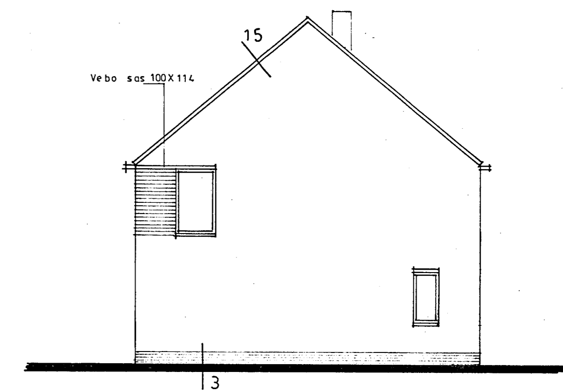
KOPGEVEL KEUKENZIJD. - beide ramen vervallen bij aansl. op garage en bij woningnrs. 37 - onderraam vervallen bij woningnrs. 7, 8, 37
