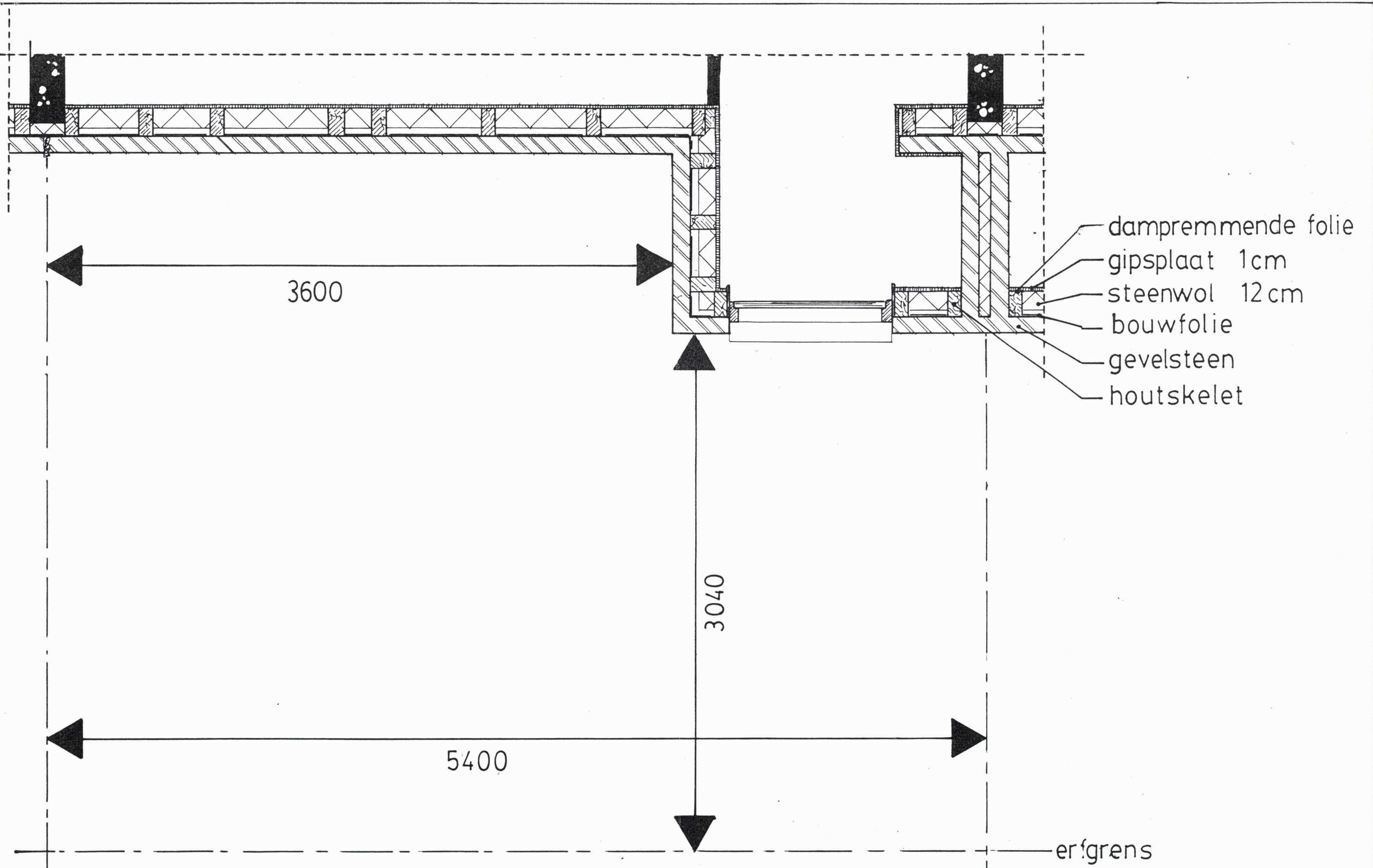
RESTMATEN VOORTUIN 1: 20
