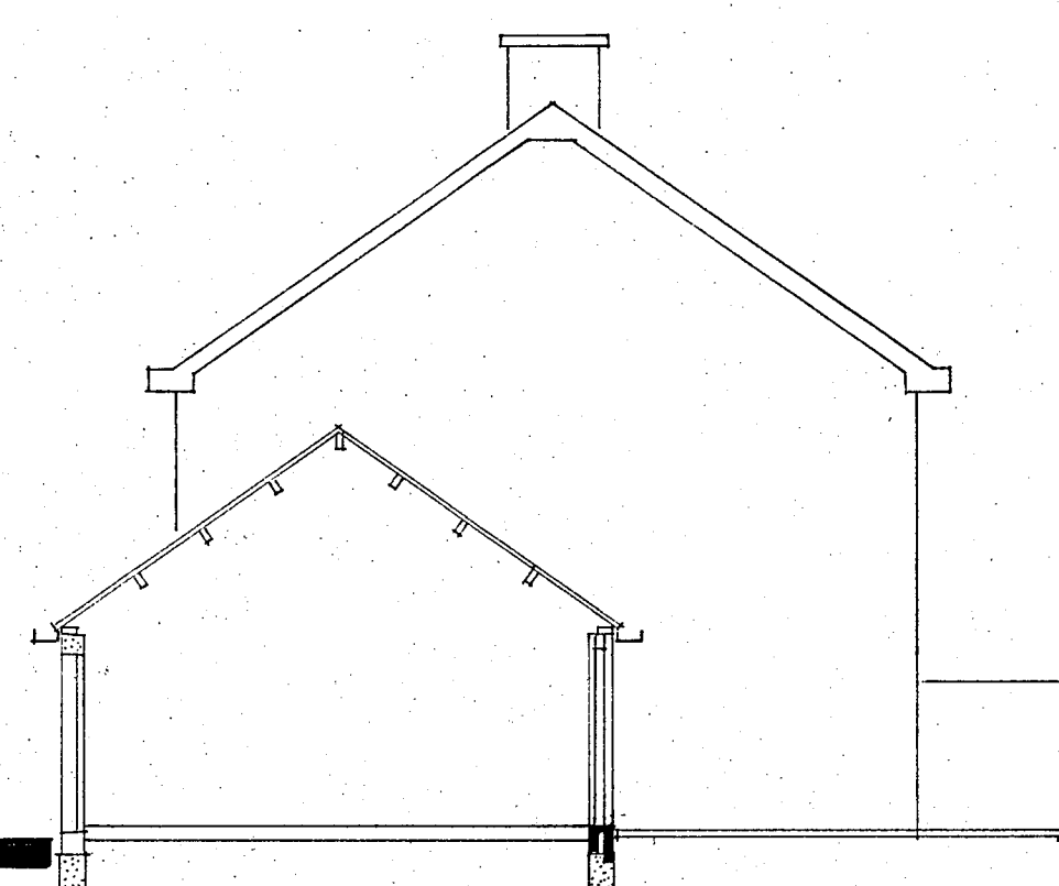
doorsnede.
