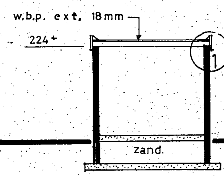
doorsnede.
