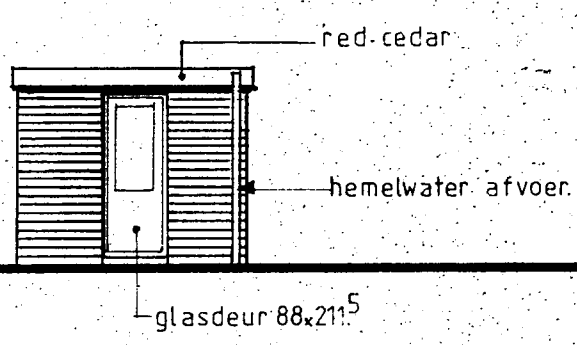
voorgevel.
