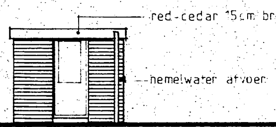
voorgevel.
