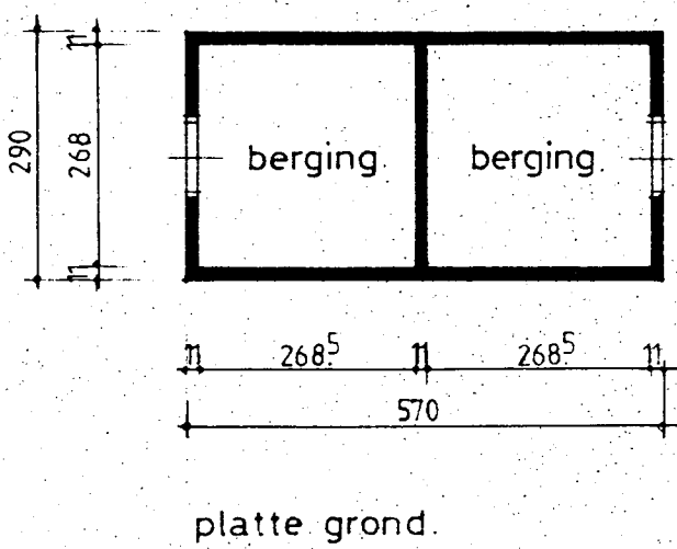
platte grond.
