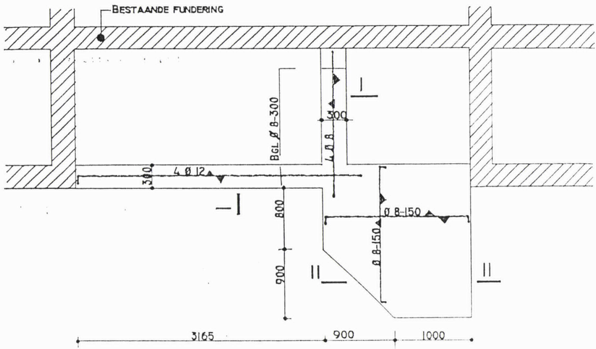
PLATTEGROND FUNDERING EN WAPENING
