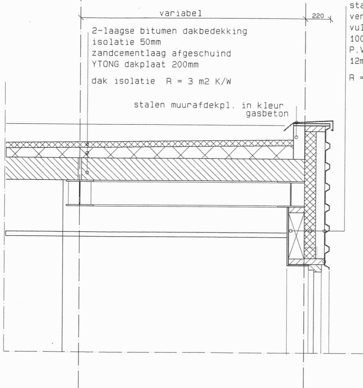
DOORSNEDE GEVEL T.P.V. BOEIDEEL
