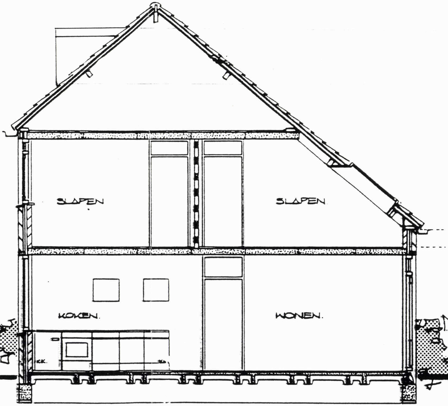
Doorsnede Type 2WA
