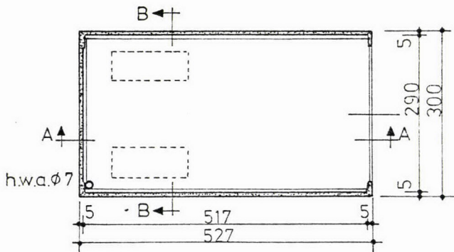
platte grond
